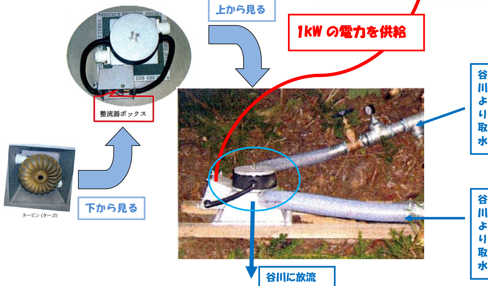
マイクロ水力発電 (ターゴインパルス型)
